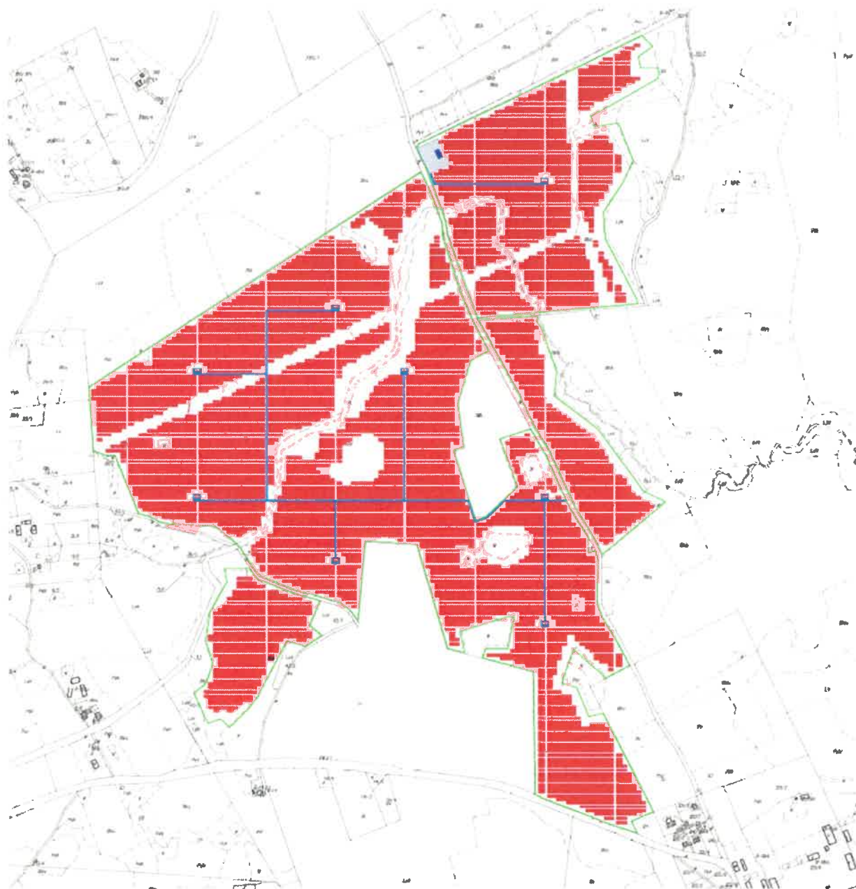
Rysunek 1 Wstępne rozmieszczenie paneli fotowoltaicznych
